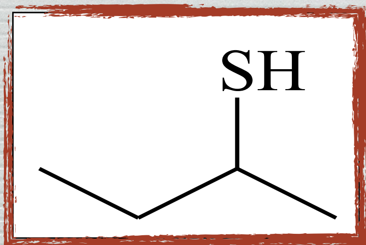
butan-2-tiol
